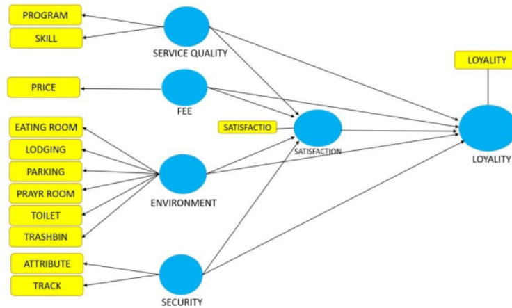
Gambar 1. Diagram Struktur Penelitian
