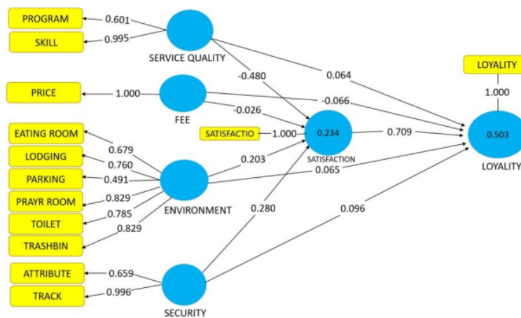
Gambar 2. Diagram Pemodelan Persamaan Struktural Hasil Penelitian
