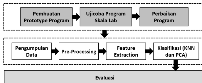
Gambar 1. Tahapan penelitian
