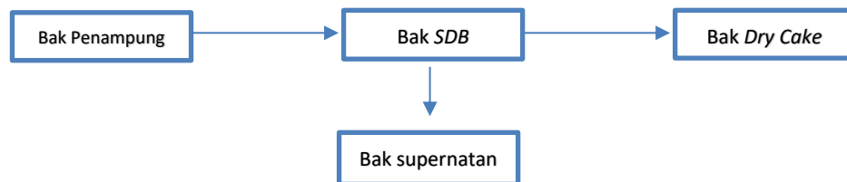
Gambar 2. Diagram Alir Pengolahan
