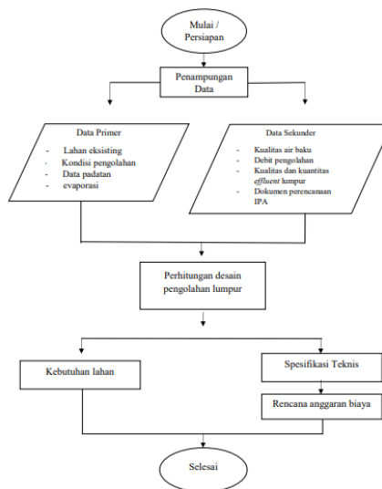
Gambar 1. Diagram Alir Perencanaan
